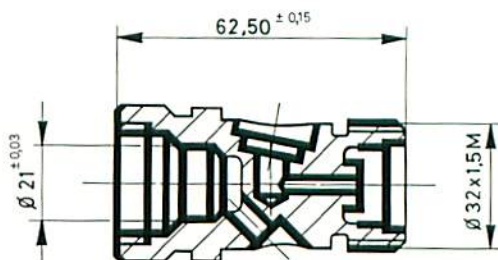
Esempio di lavorazione di particolare per regolatore pressione aria in alluminio su macchina mod. TRO-08-N 10-115-40-FMU®.
