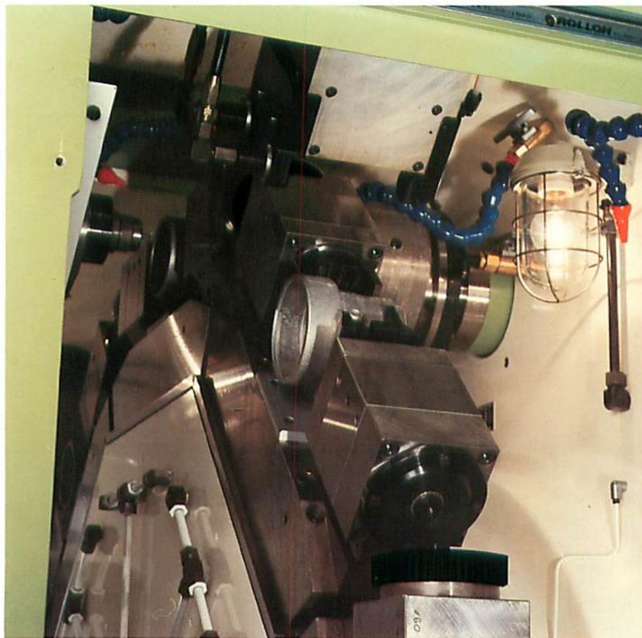
Esempio di lavorazione di particolare per regolatore pressione aria in alluminio su macchina mod. TRO-08-N 10-115-40-FMU®.
